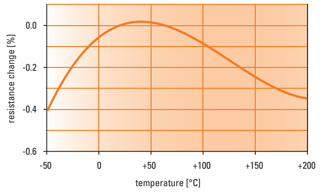
Grafik 2: Temperaturabhängigkeit des elektrischen Widerstands (-50 °C bis +200 °C)
